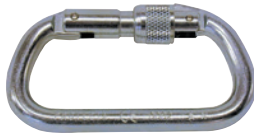
Mousqueton à vis type PRAJ501 Ouverture 17 mm. Résistance 25 KN. Conforme EN 362.
